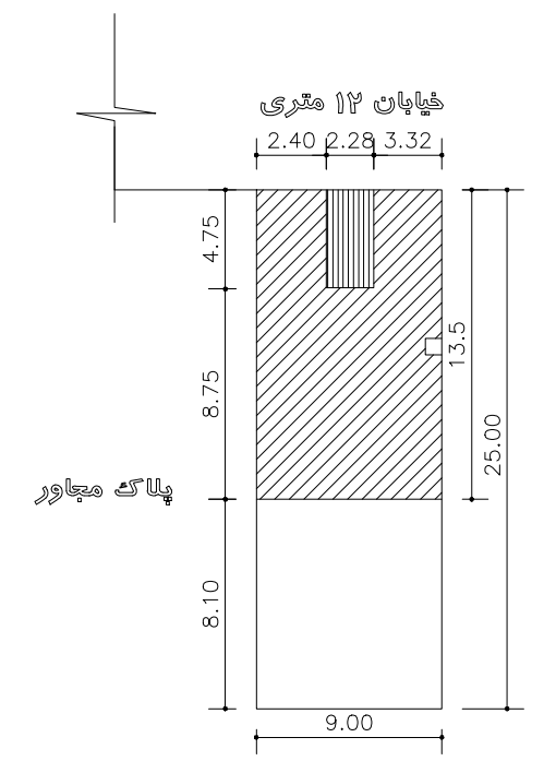
پلاک مجاور پلان موقعیت SC 1/100
