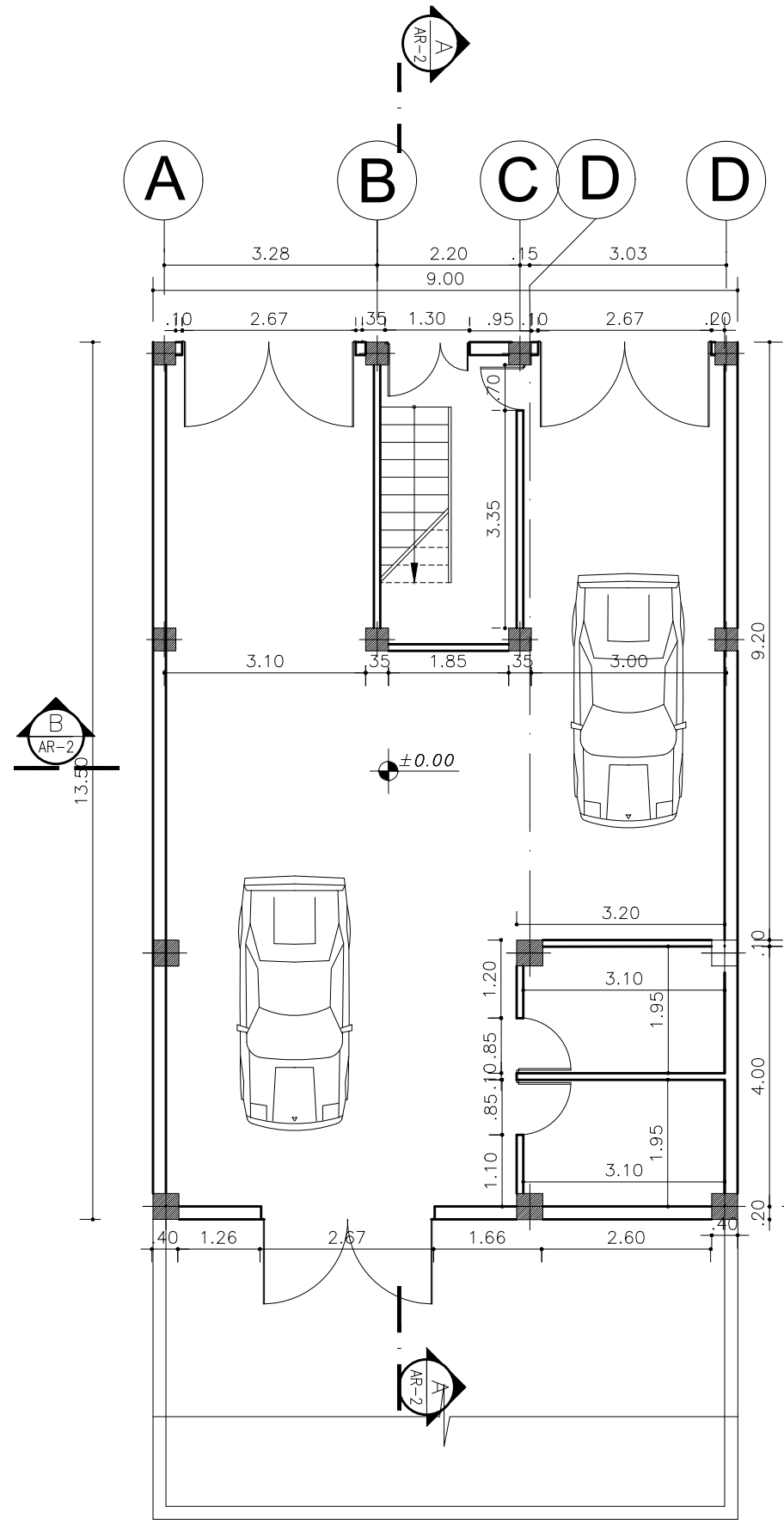
پلان طبقه همکف SC 1/100
